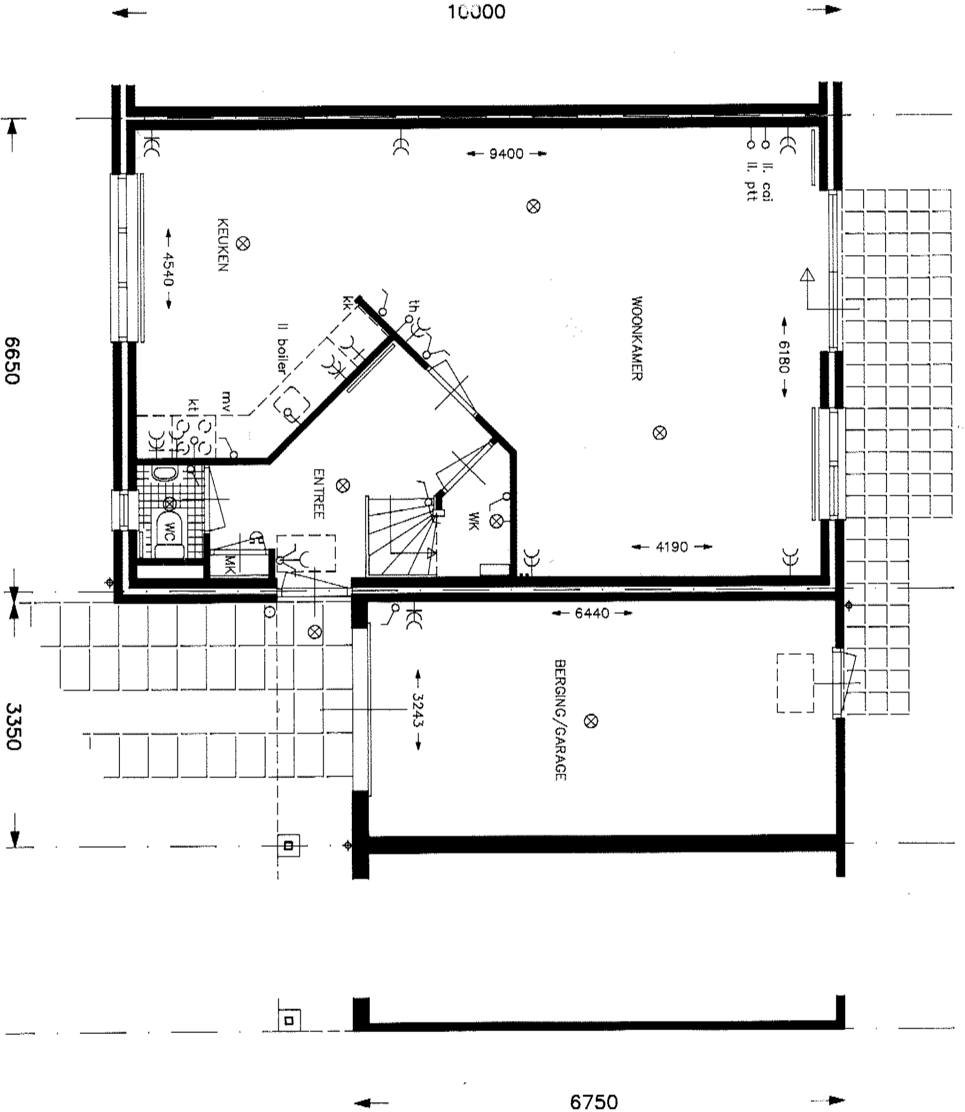
Begane grond type F1 standaard
