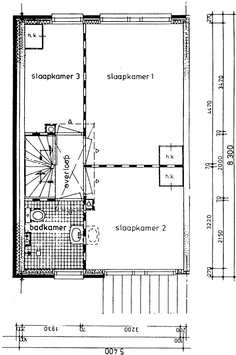
1 e verdieping type A
