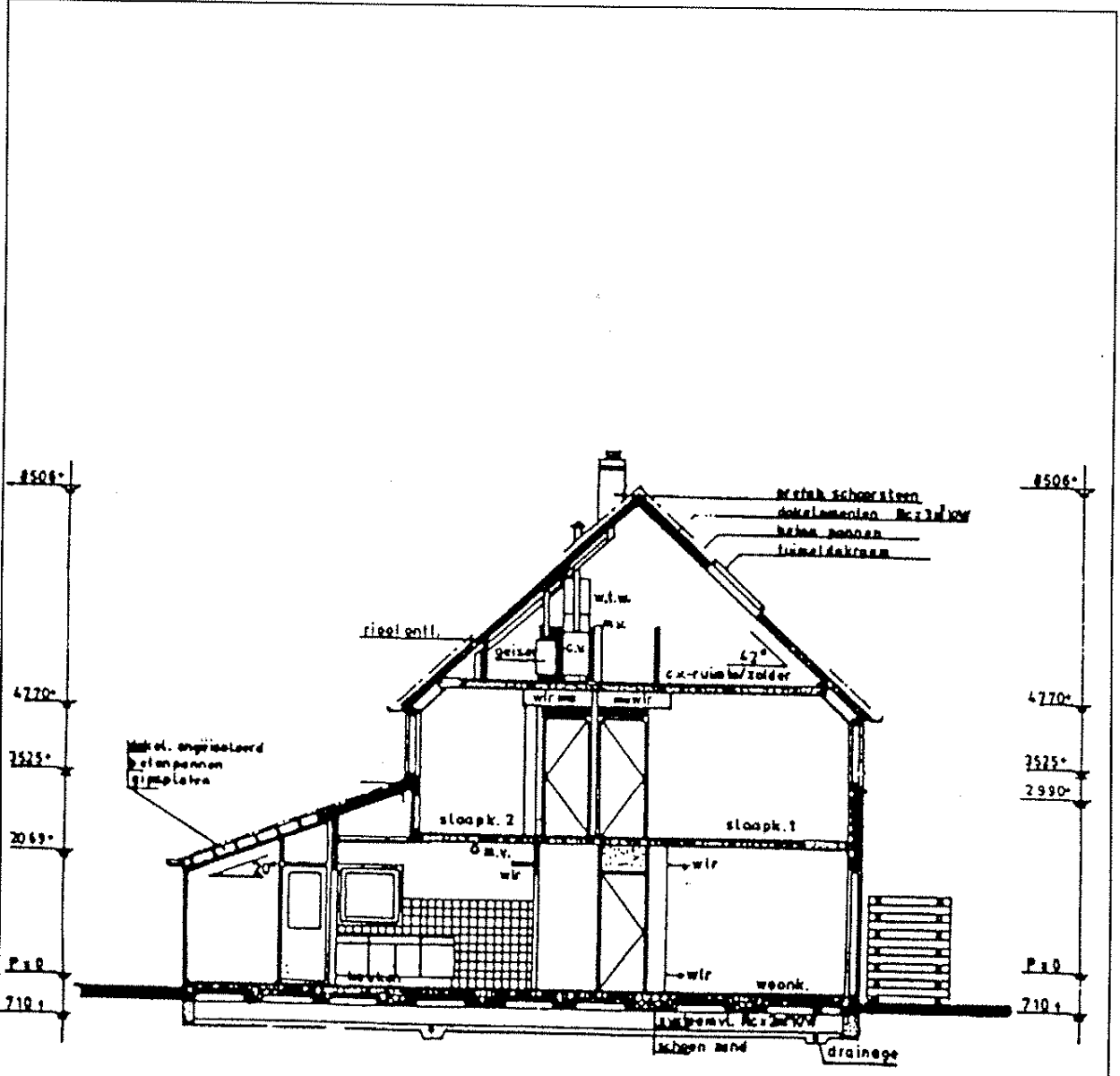
— doorsnede type A —
