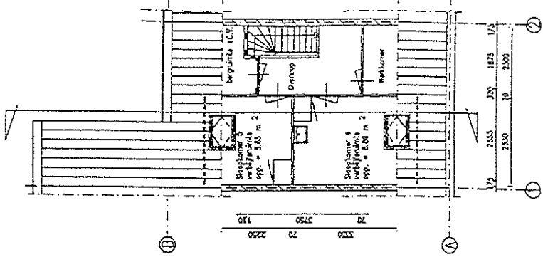
Plattegrond (2e verd.)
