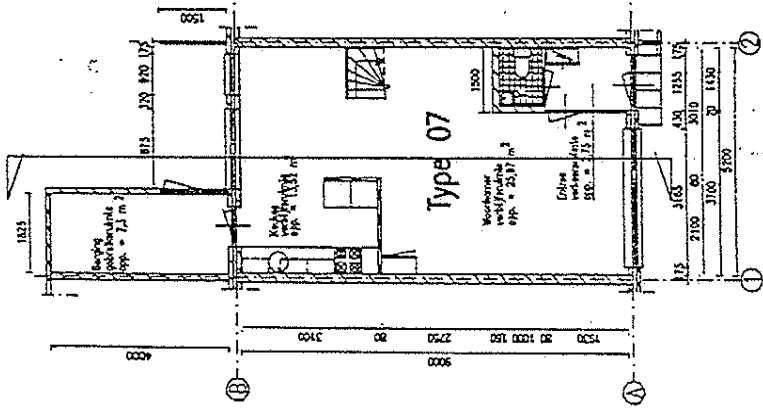
Plattegrond (beg.gr.)
