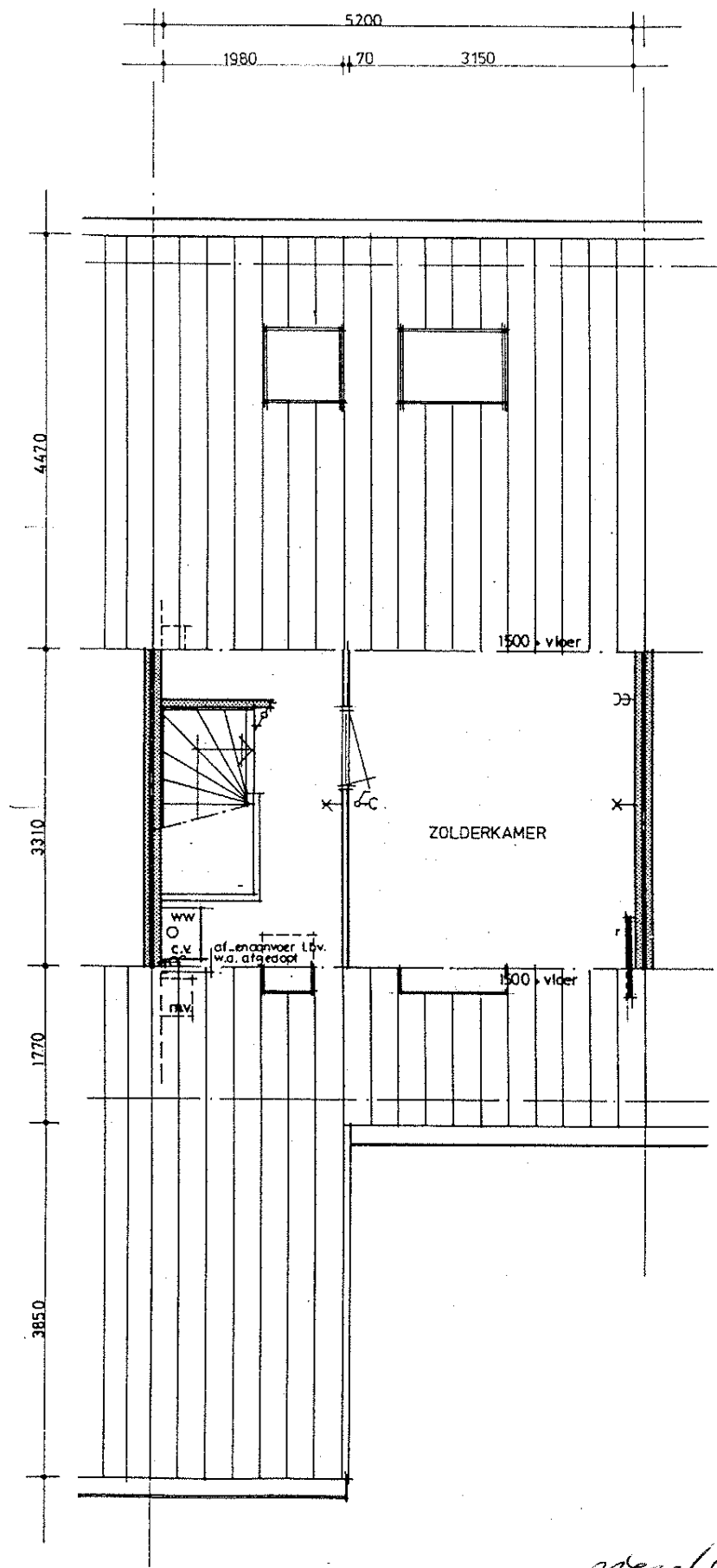
VERDIEPING 5400. (variant 4 = zolderkamer + dakraam.)
