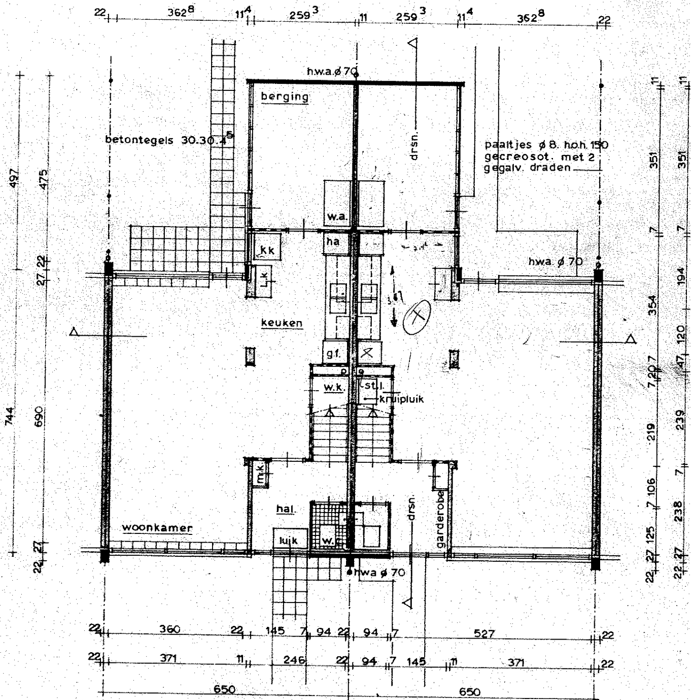
plattegrond begane_grond
