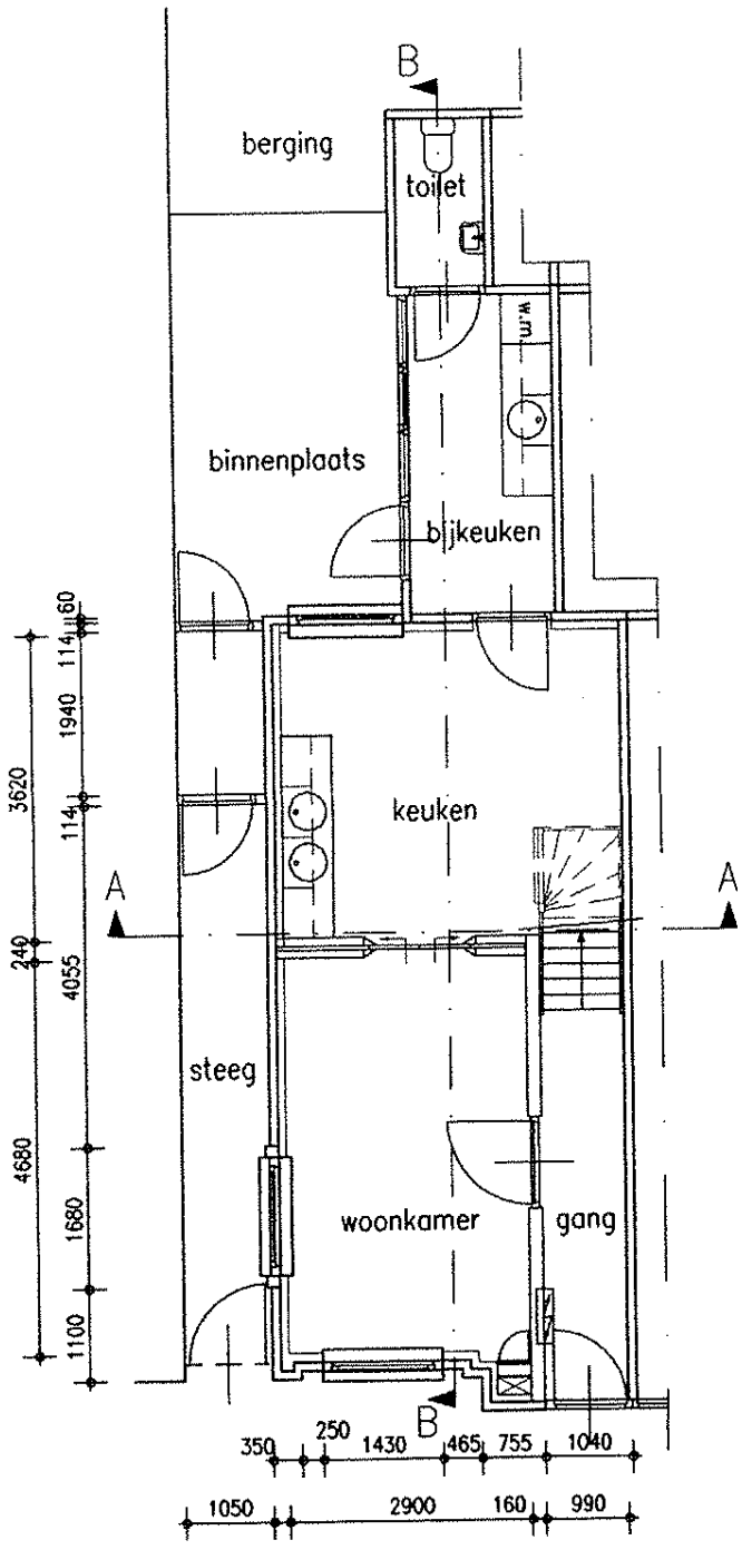
Begane grond
